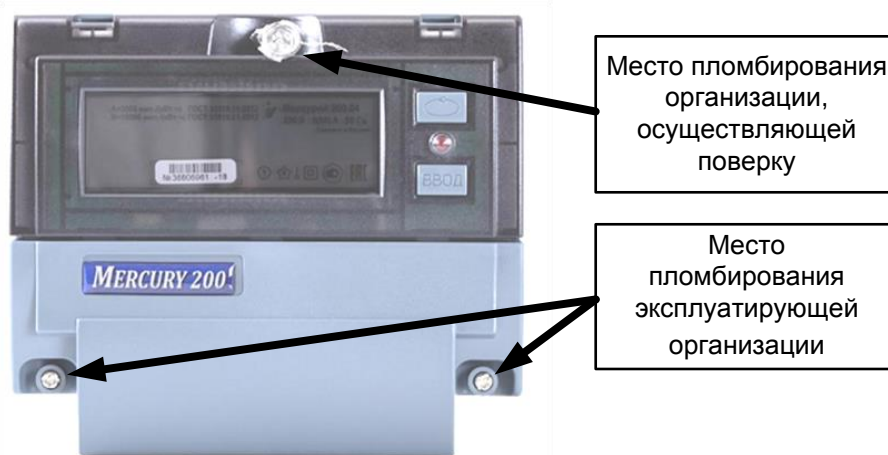
Рисунок 2.1 – Схема пломбирования
