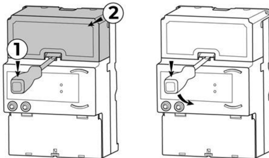
Рисунок 6.4 – Доступ к сменному модулю связи
