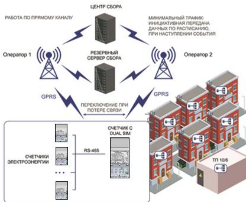
Рисунок 5.3 – Схема работы счетчика DUAL SIM в составе АИИС КУЭ
