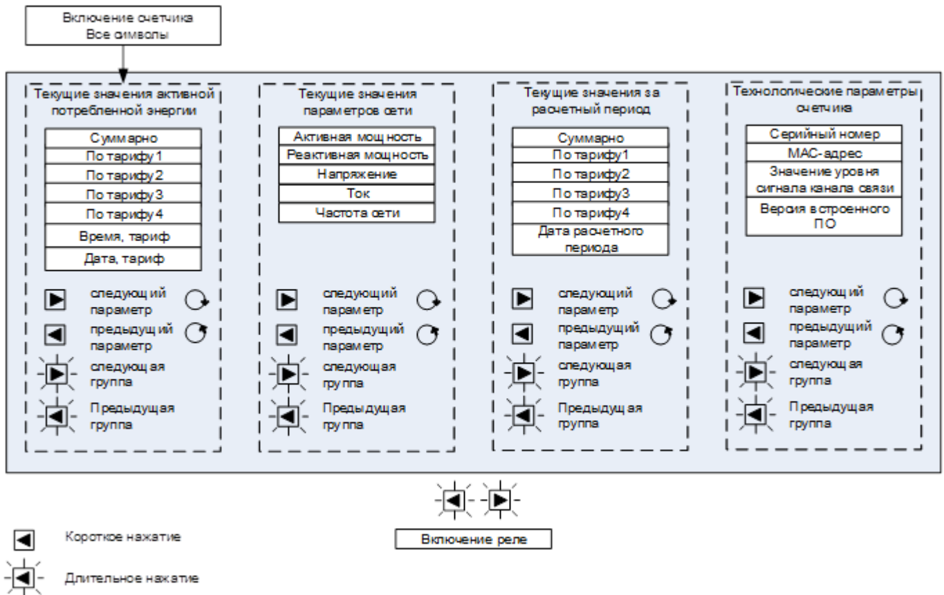
Рисунок 6.7 – Группы индикации по умолчанию и переходы между ними
