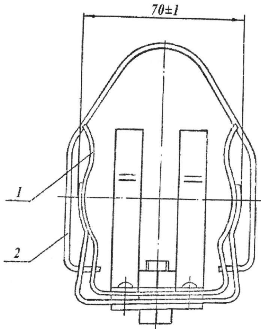
Рис. 1. Контакт предохранителя серии ПКТ 102-103: 1 – губка контактная; 2 – замок. 1
