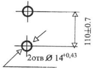
Разметка отверстий под установку предохранителей серий:ПКТ 101-6; ПКТ 101-10 ПКН 001-10У1
