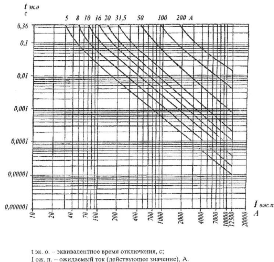
Рис. 3. Время-токовые характеристики отключения предохранителей типоразмеров с порядковыми номерами по таблице 1 — 18, 30-34, 46, 60, 68 на номинальные токи 5-31,5, 50, 100А.
