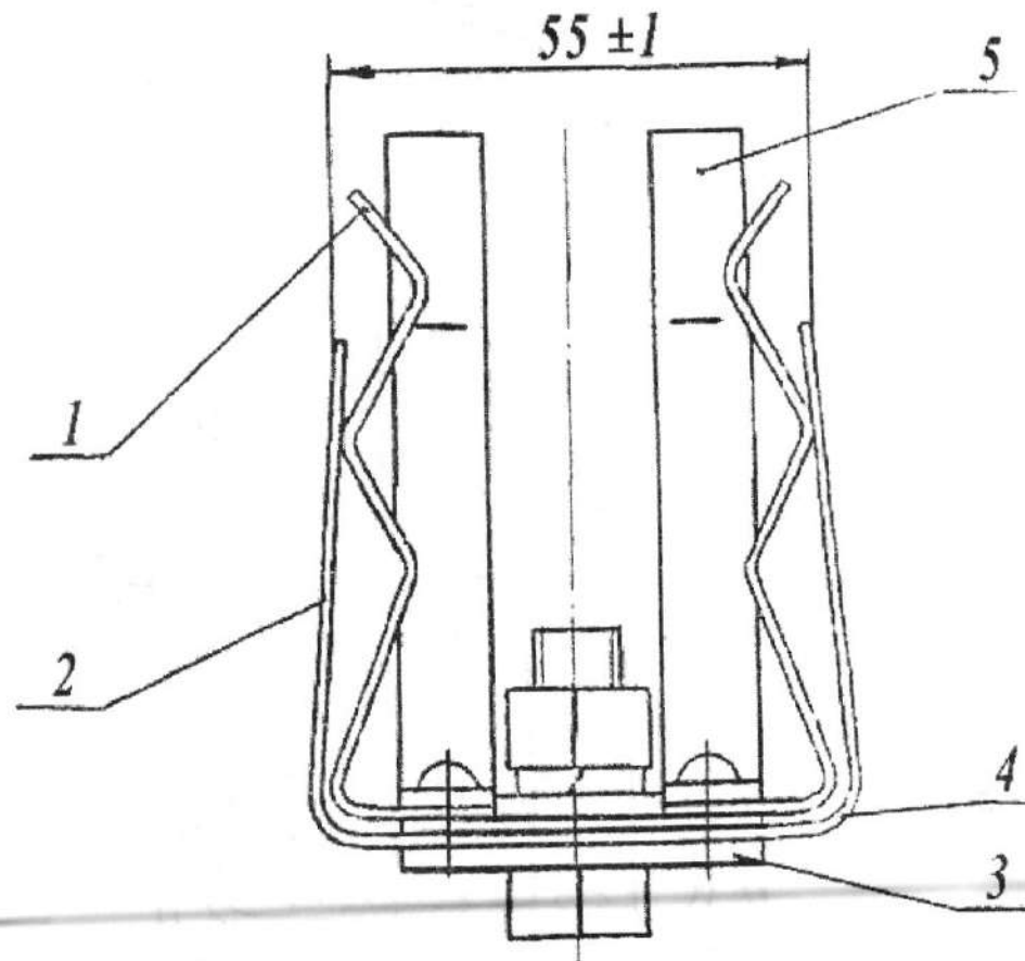
Рис. 1. Контакт предохранителя серии ПКТ 101: 1 — губка контактная; 2 — скоба; 3 — планка стальная; 4 — планка медная; 5 — ограничитель. 1
