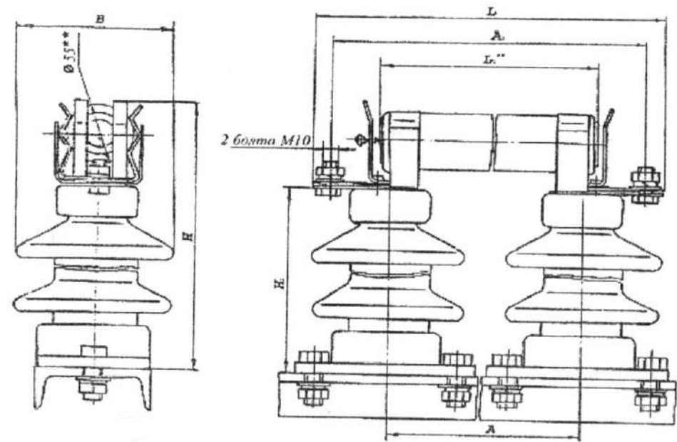
Разметка отверстий под установку предохранителей серий:ПКТ 101-6; ПКТ 101-10 ПКН 001-10У1
